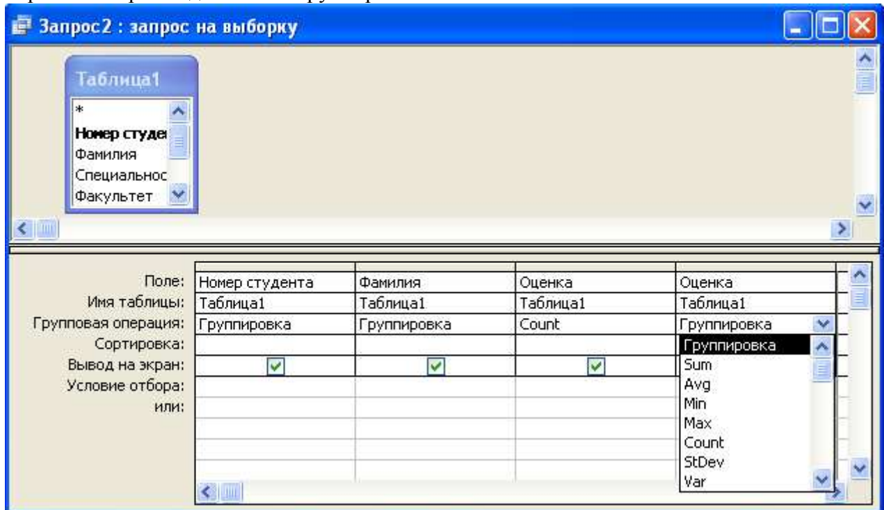
Рис. 19. Структура запроса на группирование данных
